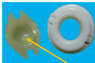
قطعه کائوچونی نصب شده بر روی دوشاخه کلاچ ۱۸۱۰۷۰۷۸
