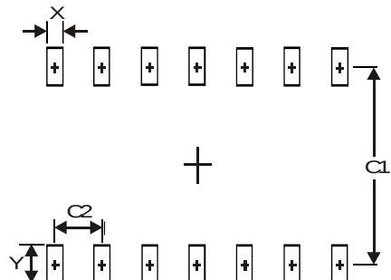
SO-14
